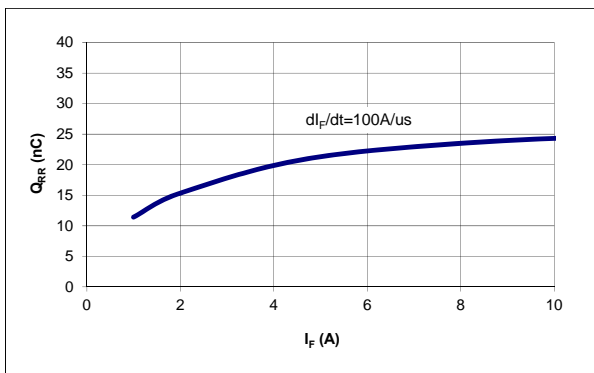
图7. 典型 Q_{RR} 与 I_F 比较, T_J = 125\text{ }^\circ\text{C}
