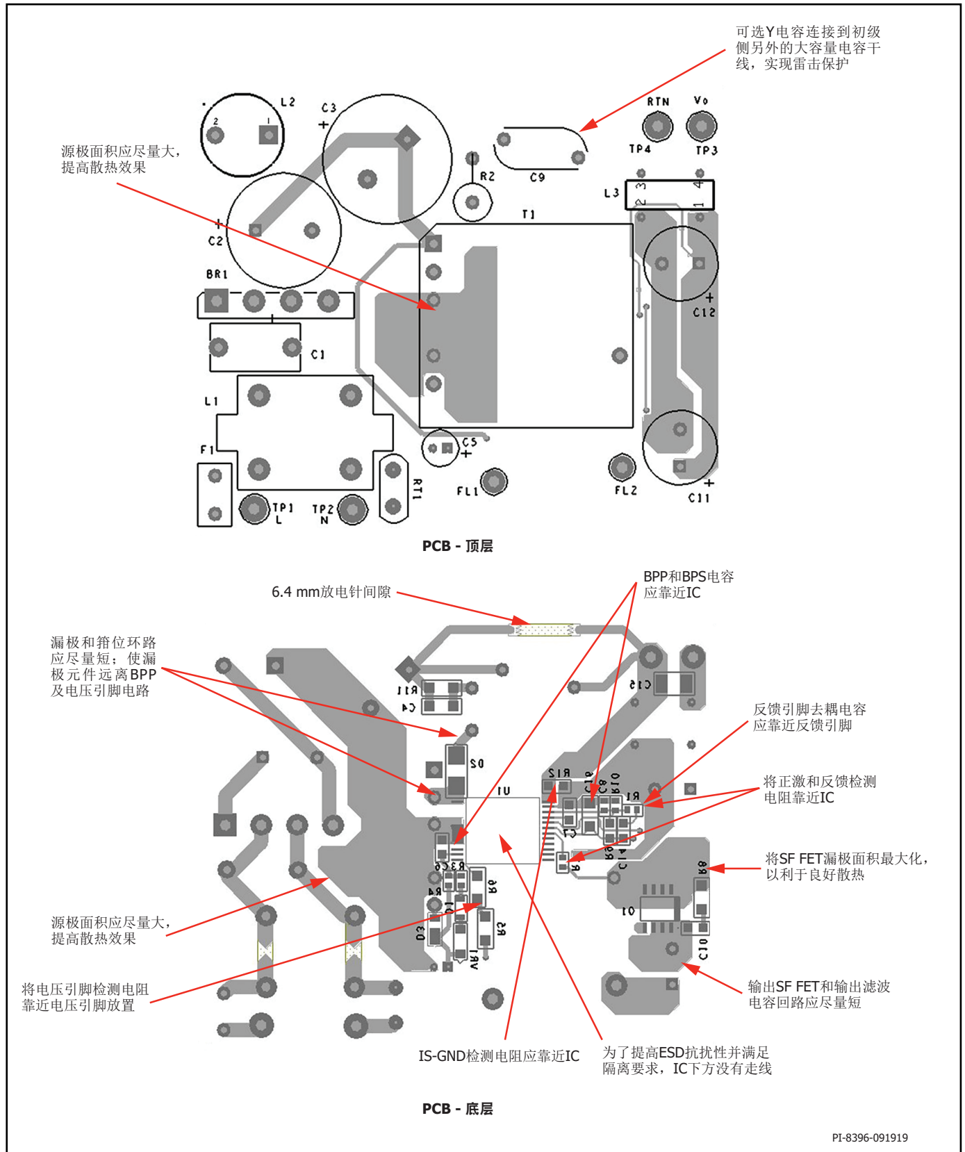
图18. PCB
