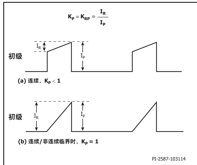
图19. 连续导通模式电流波形, K_p < 1
