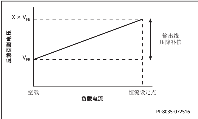
图8. 输出线压降补偿特性
