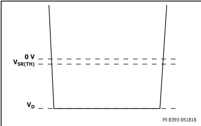
图15. 握手前反激周期中体二极管导通期间可接受的正激引脚电压波形
