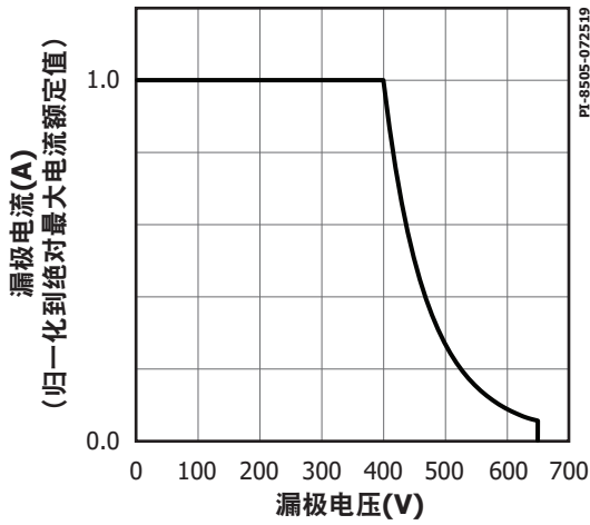
图21. 最大允许的漏极电流相对于漏极电压的变化
