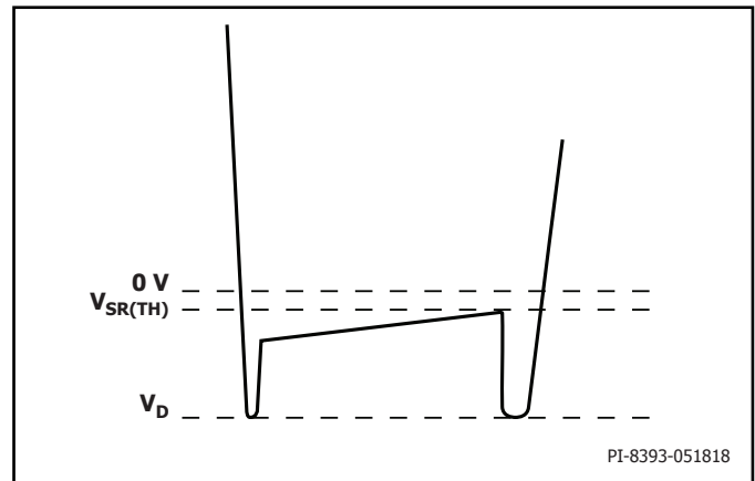
图13. 握手后反激周期中SR开关导通期间可接受的正激引脚电压波形
