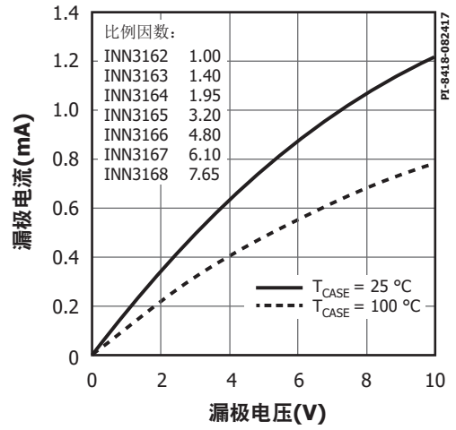
图22. 输出特性
