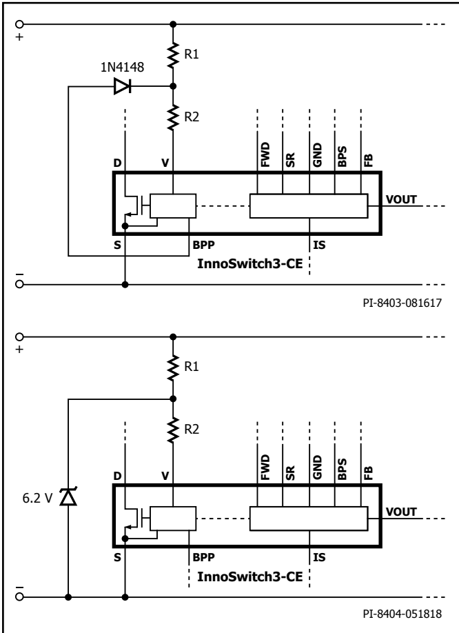
图16. (顶部) 仅使能输入过压保护; (底部) 仅使能输入欠压保护
