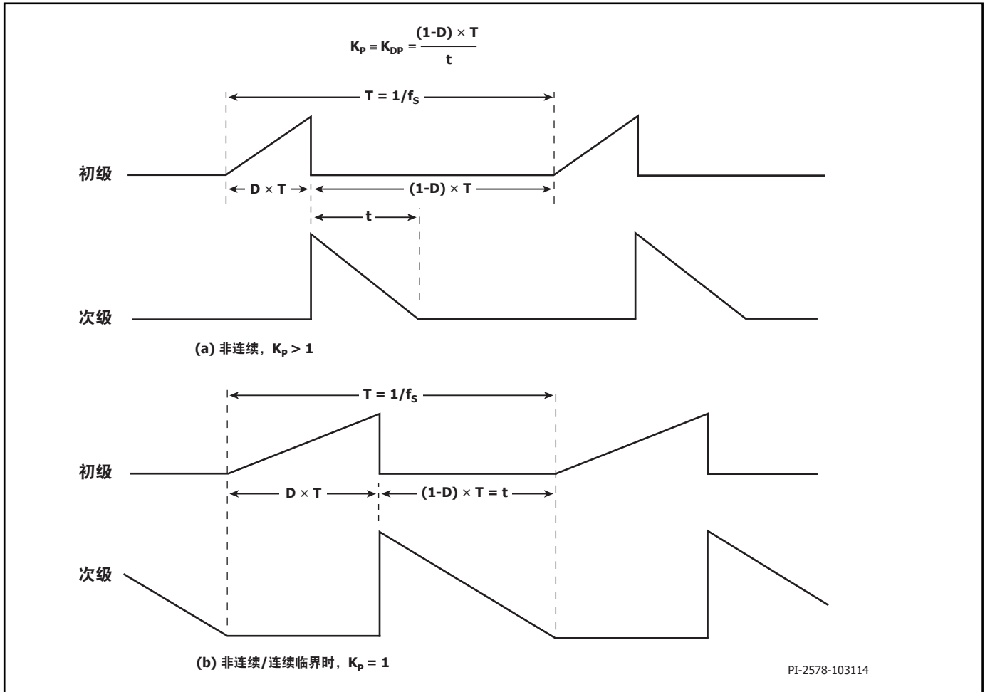
图20. 非连续导通模式电流波形, K_p > 1
