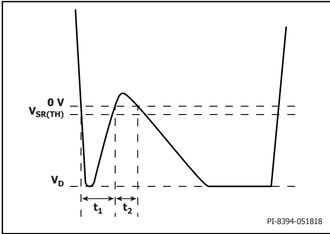
图14. 握手前反激周期中体二极管导通期间不可接受的正激引脚电压波形 注:
