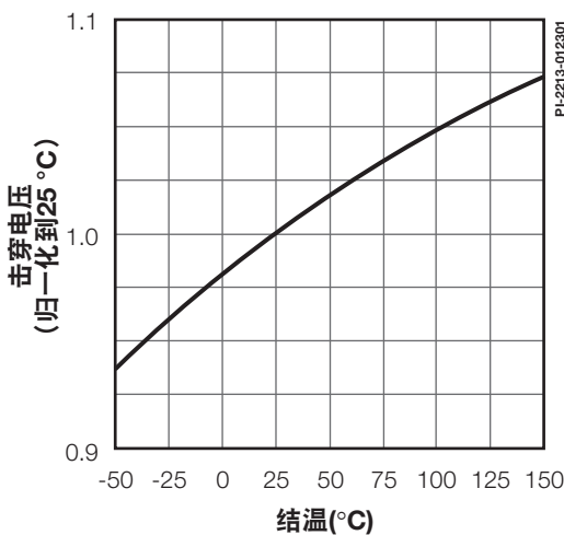
图25. 击穿电压相对于温度的变化
