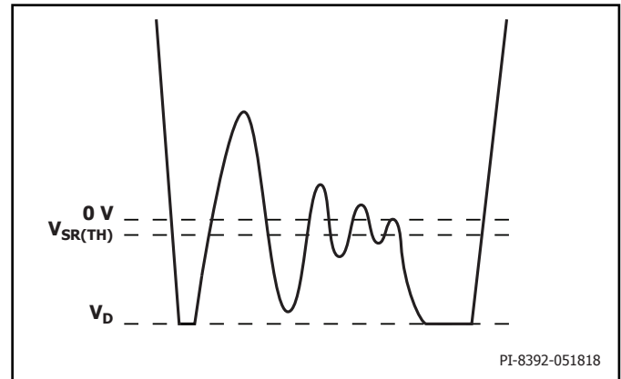
图12. 握手后反激周期中SR开关导通期间不可接受的正激引脚电压波形
