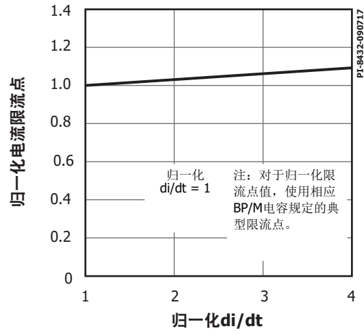
图27. 标准限流点相对于di/dt的变化
