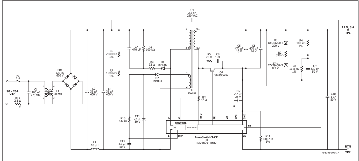
图11. 12 V/3 A充电器/适配器
